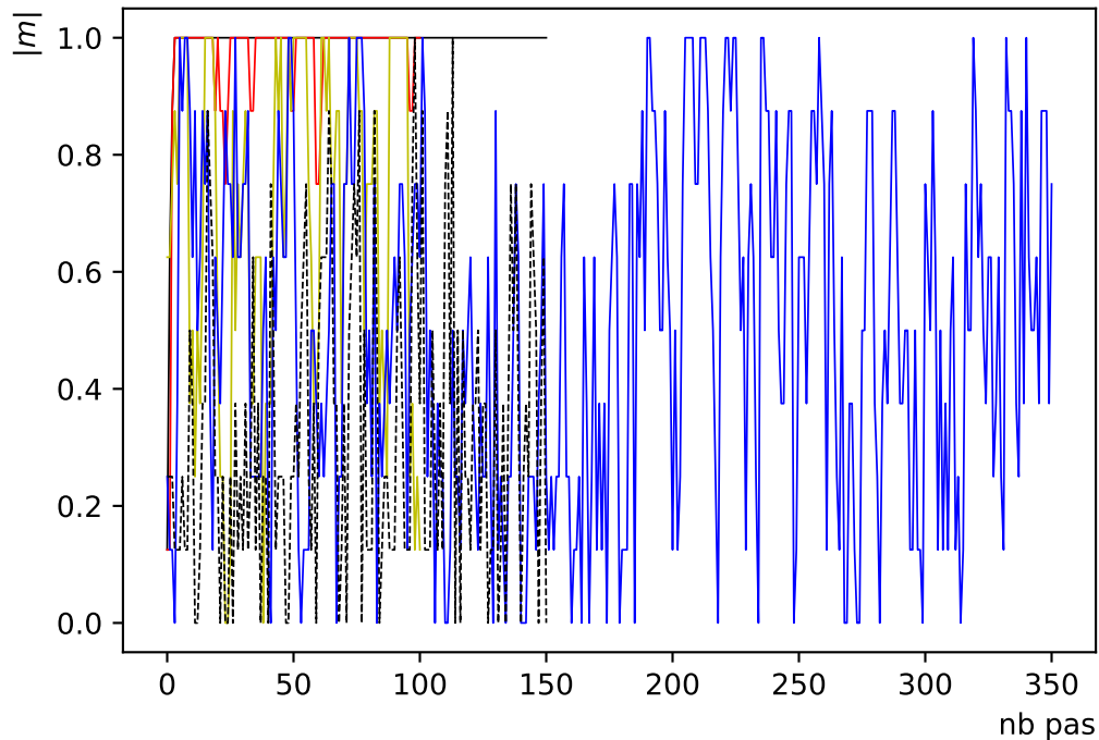
Evolution selon critère Estimation par intervalle,Condition Initiale aléatoire de taille L=4
